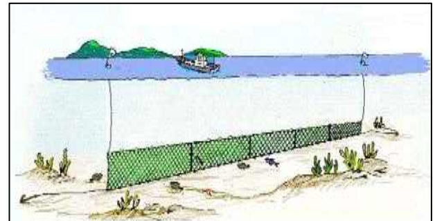
<자망(고정) 조업모식도>
